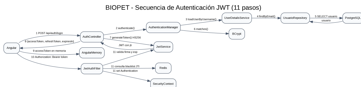
Figura 3: Diagrama de secuencia de la autenticación JWT.
