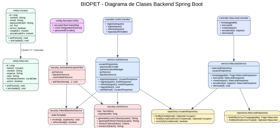
Figura 2: Diagrama de clases del backend Spring Boot.
